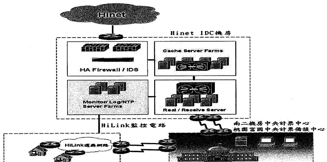
圖 2、網路規畫圖
