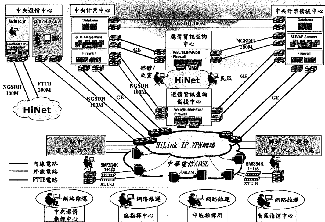
圖 1、計票系統網路規畫圖
